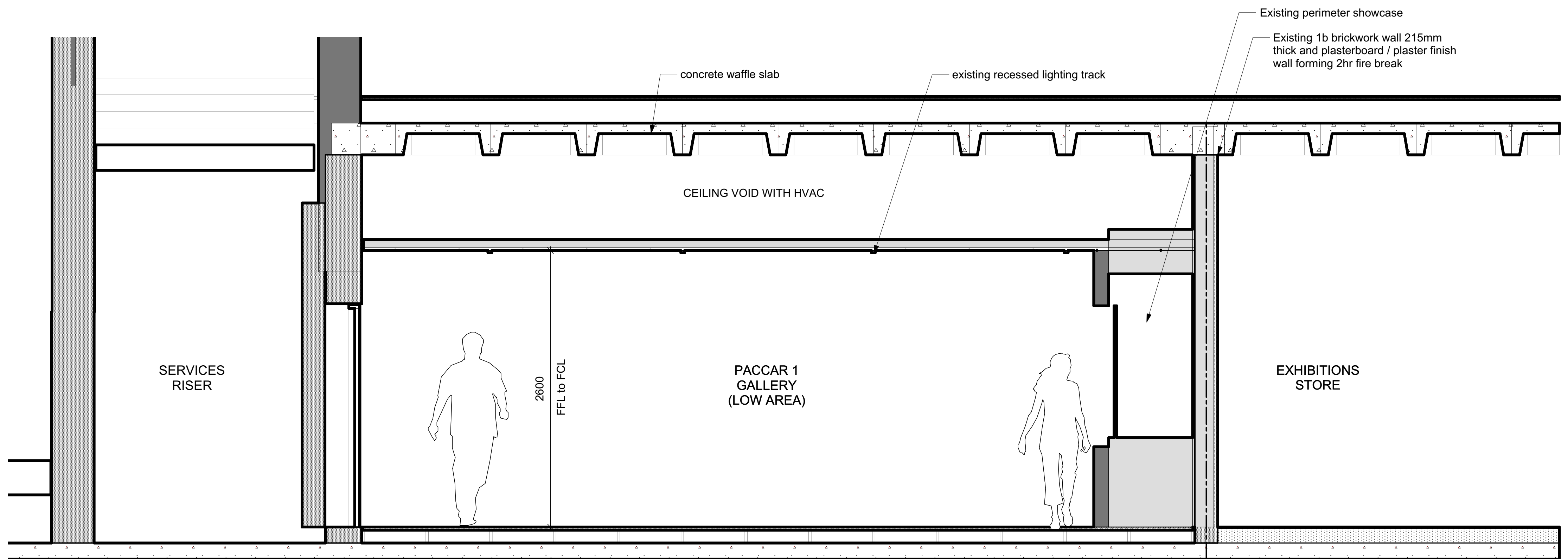
2 Section J-J Scale: 1:25
