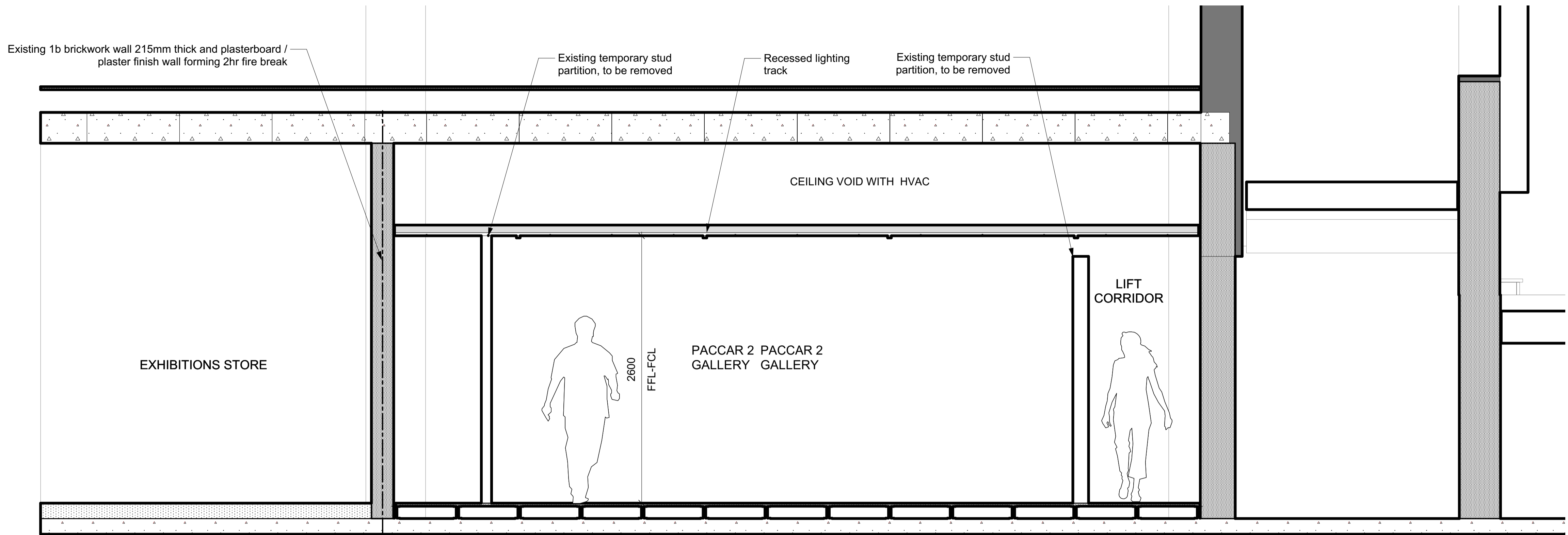
2 Section G-G Scale: 1:25
