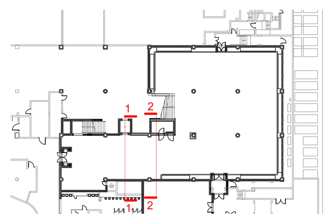
3 KEYPLAN Scale: 1:400
