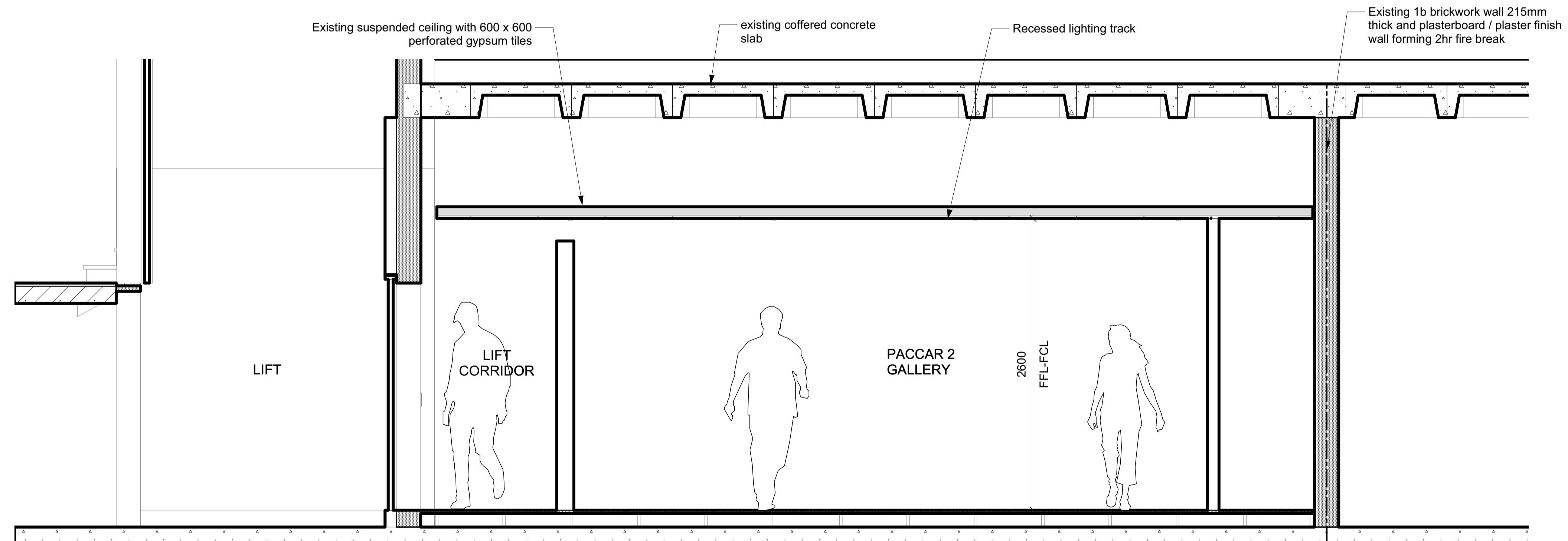
1 Section H-H Scale: 1:25
