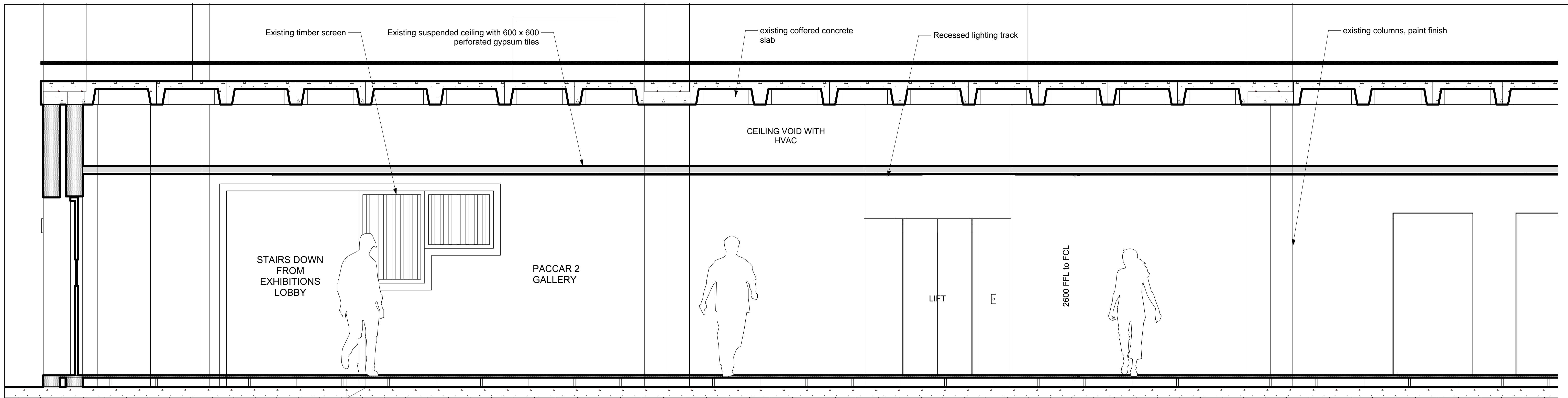
1 Section A-A Scale: 1:25
