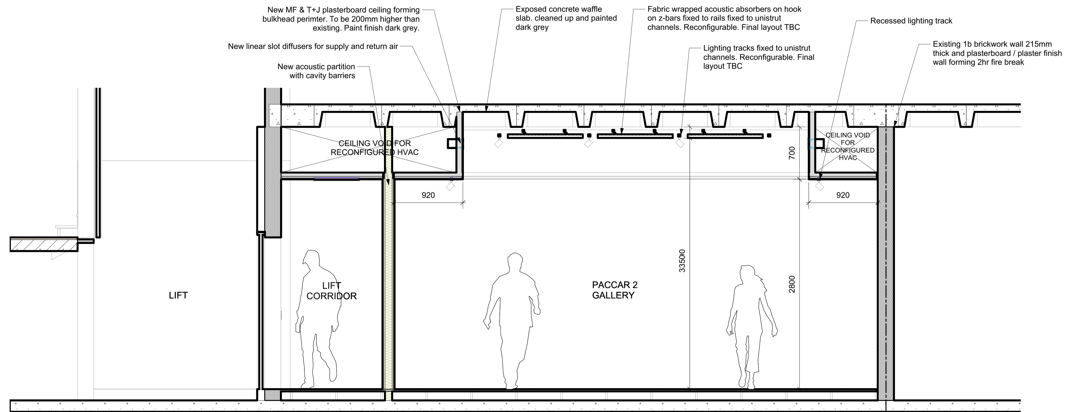
1 Section H-H Scale: 1:25
