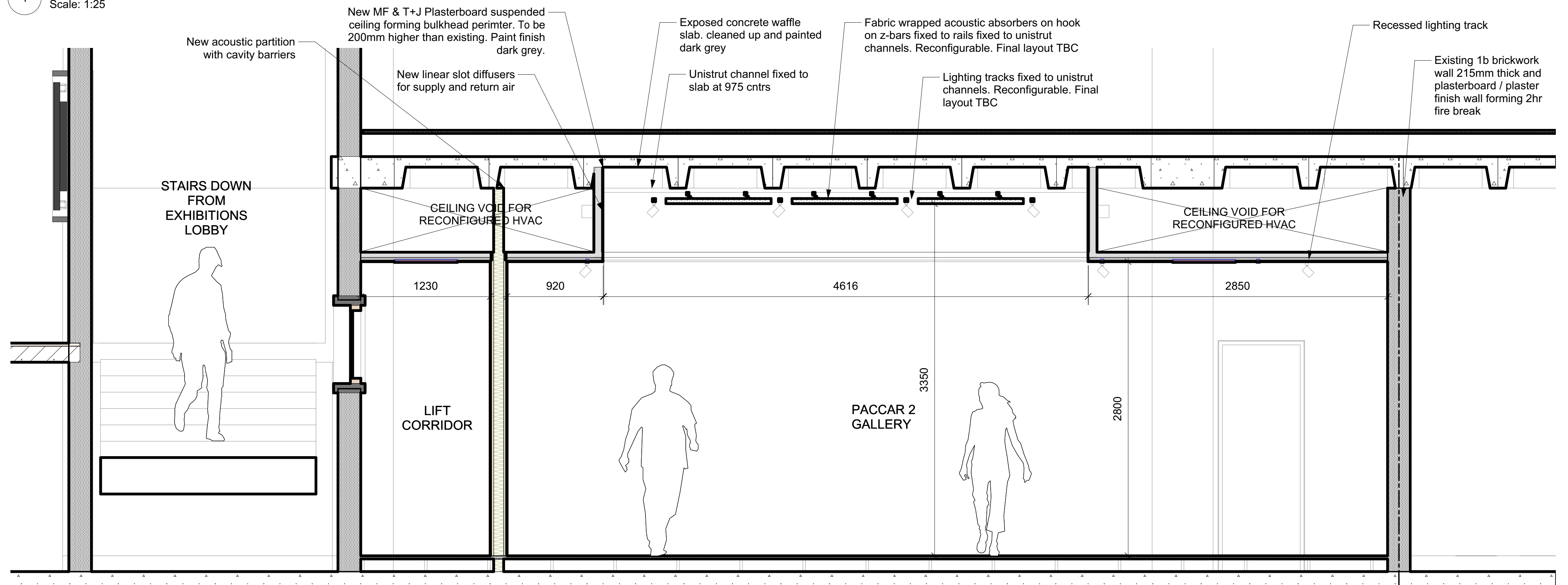
2 Section F-F Scale: 1:25
