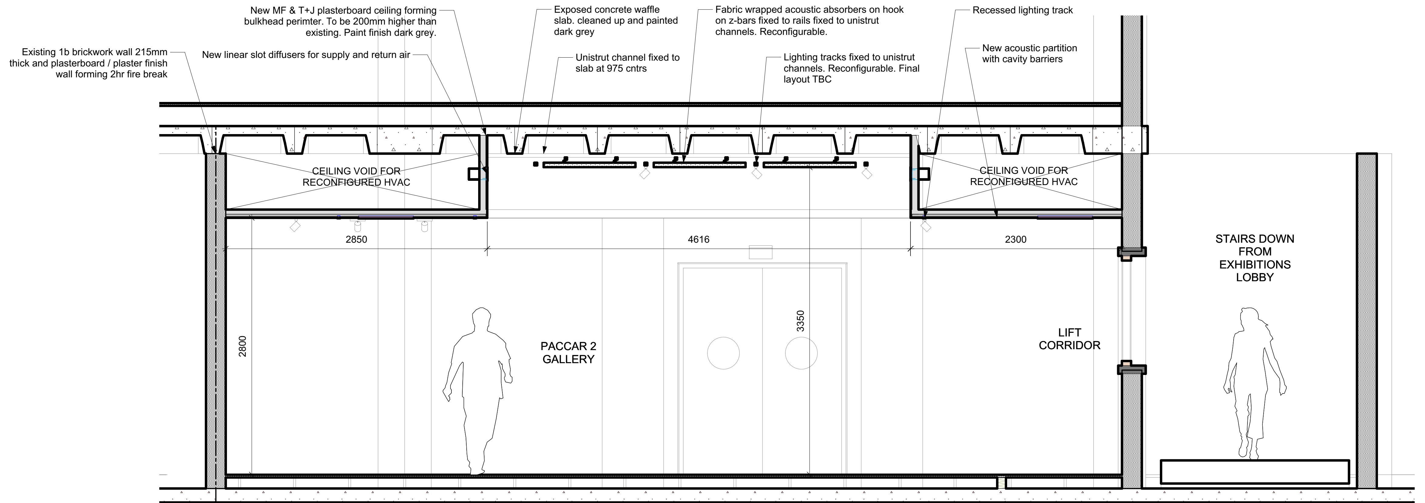
1 Section E-E Scale: 1:25
