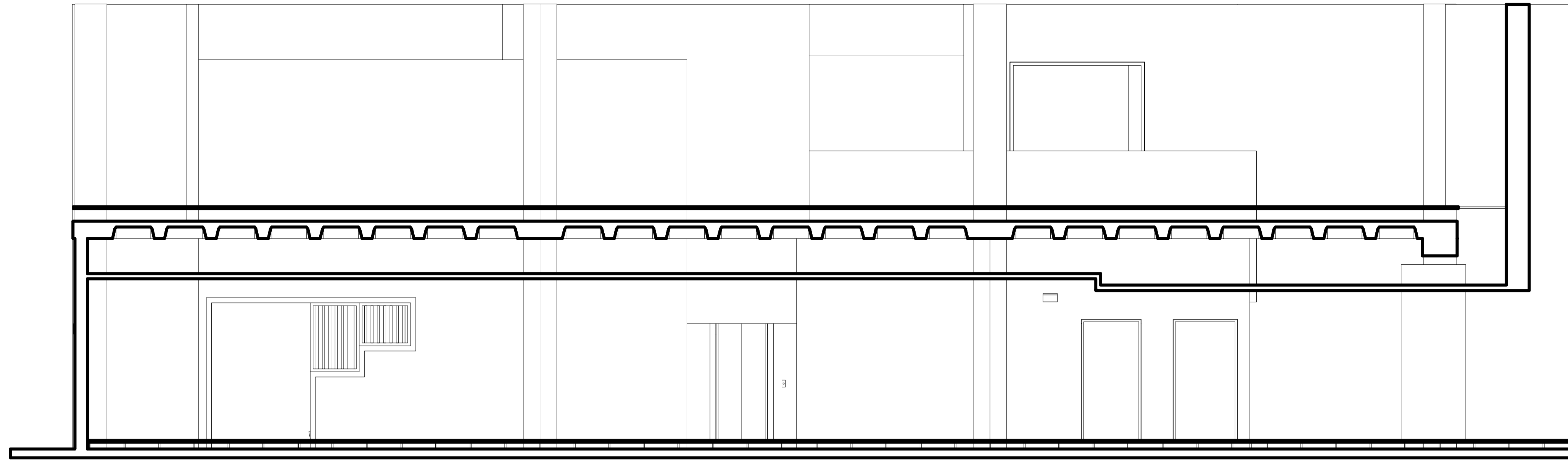
1 Section C-C Scale: 1:50
