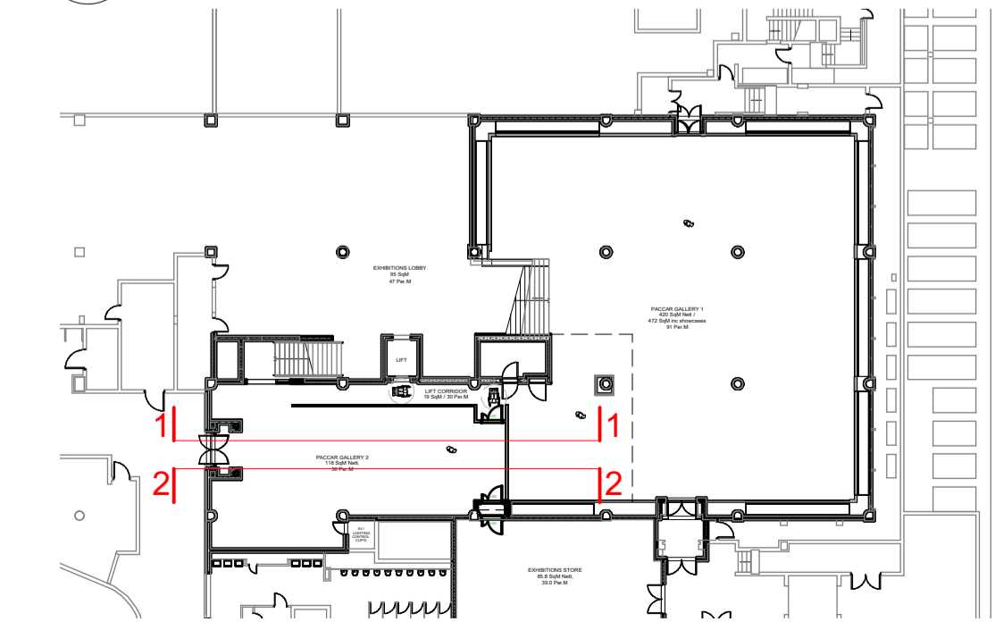
3 KEYPLAN Scale: 1:400
