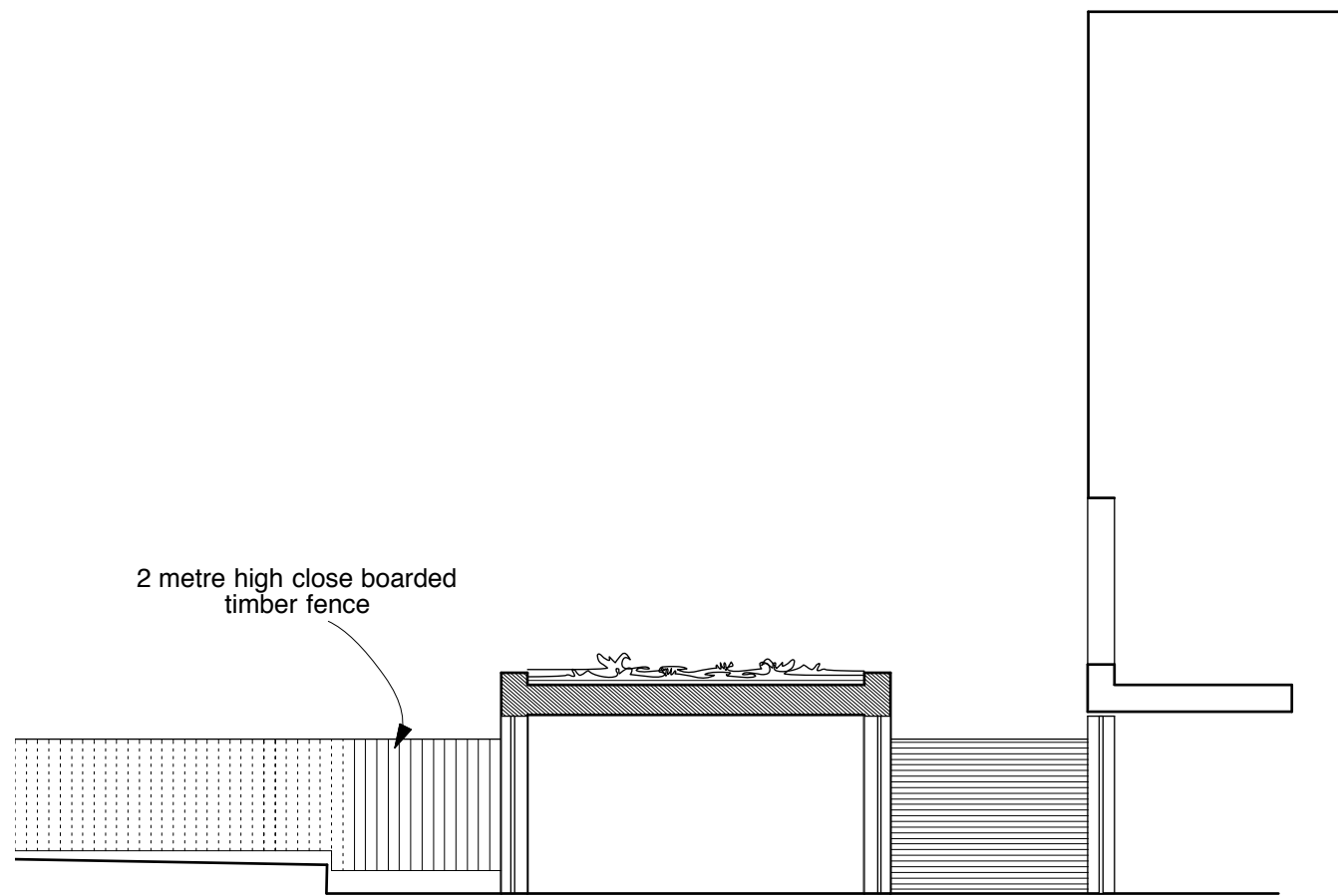
section dd
