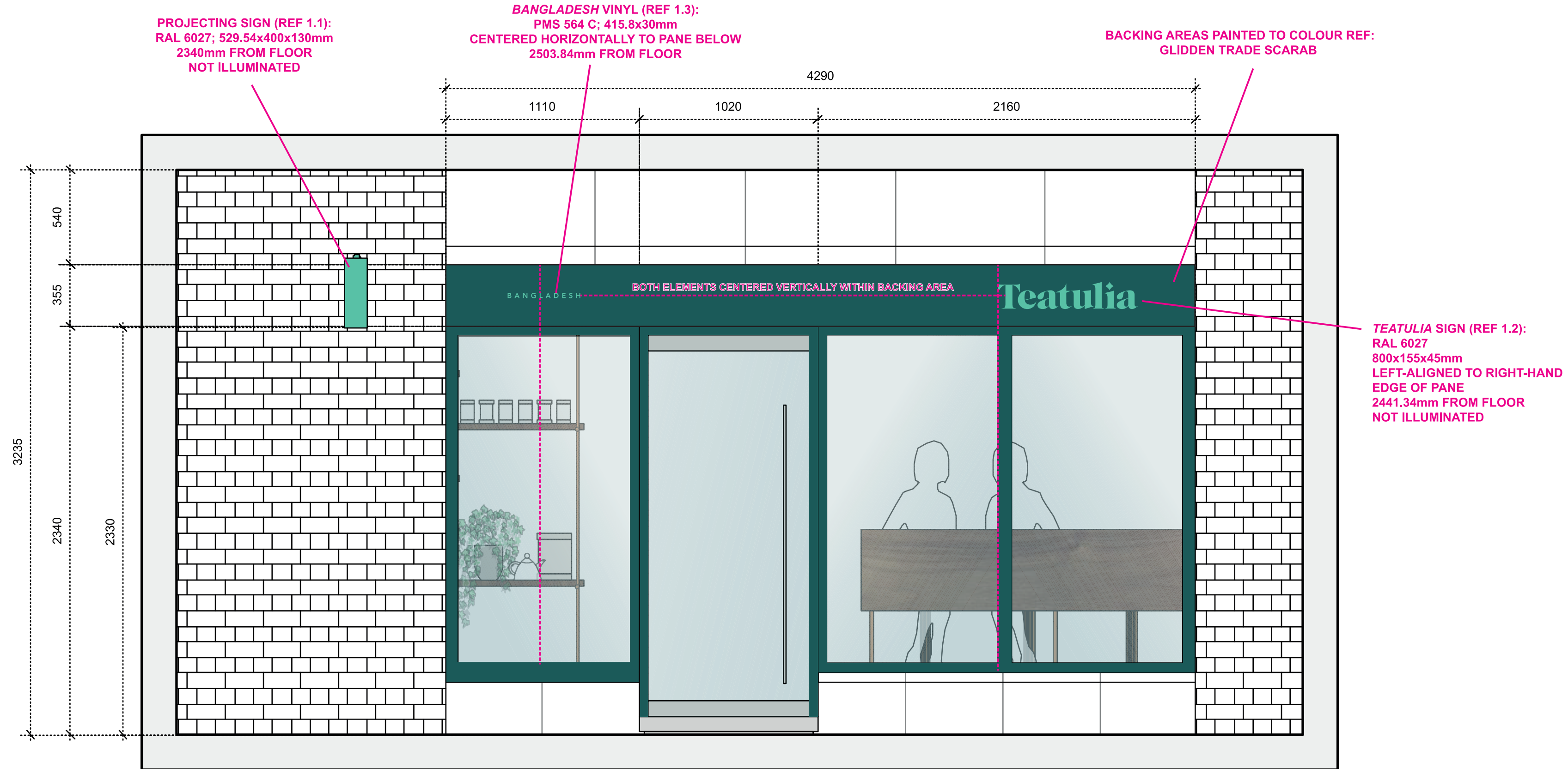
1 SE-05 EXTERIOR ELEVATION Scale: 1:20
