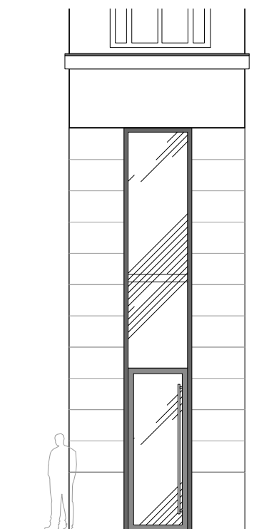
03 ELEVATION C 1:50 @ A1 1:100 @ A3
