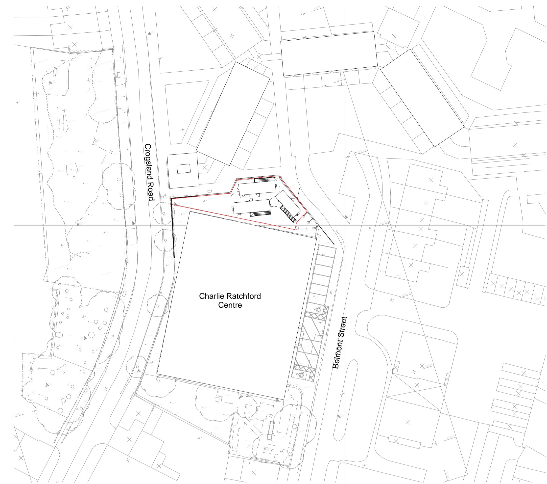
Site Plan 1:500
