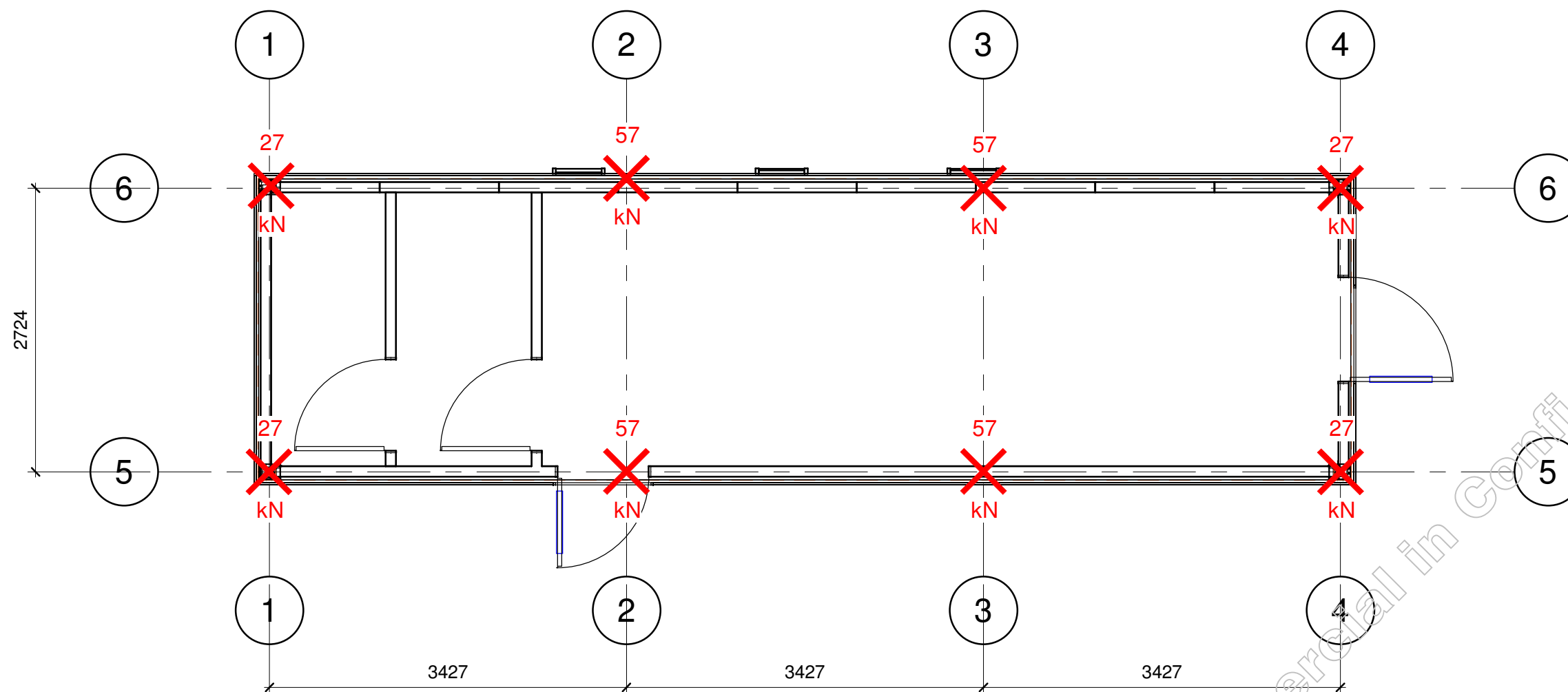
1 Level 0 FO 1 : 50
