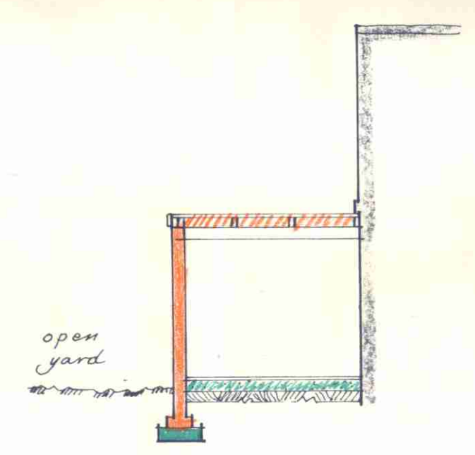
SECTION D-D
