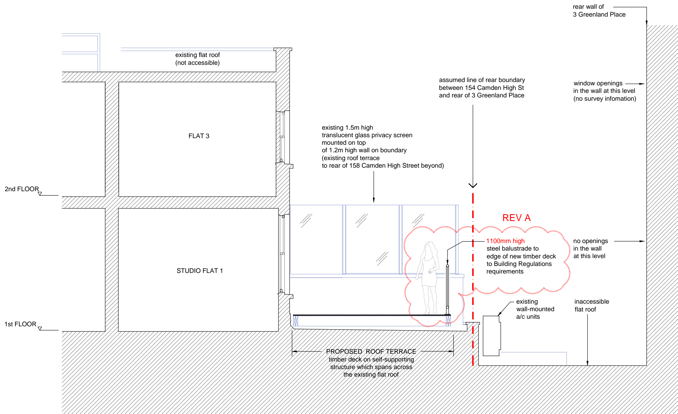
SECTION D-D 1:50 @ A3
