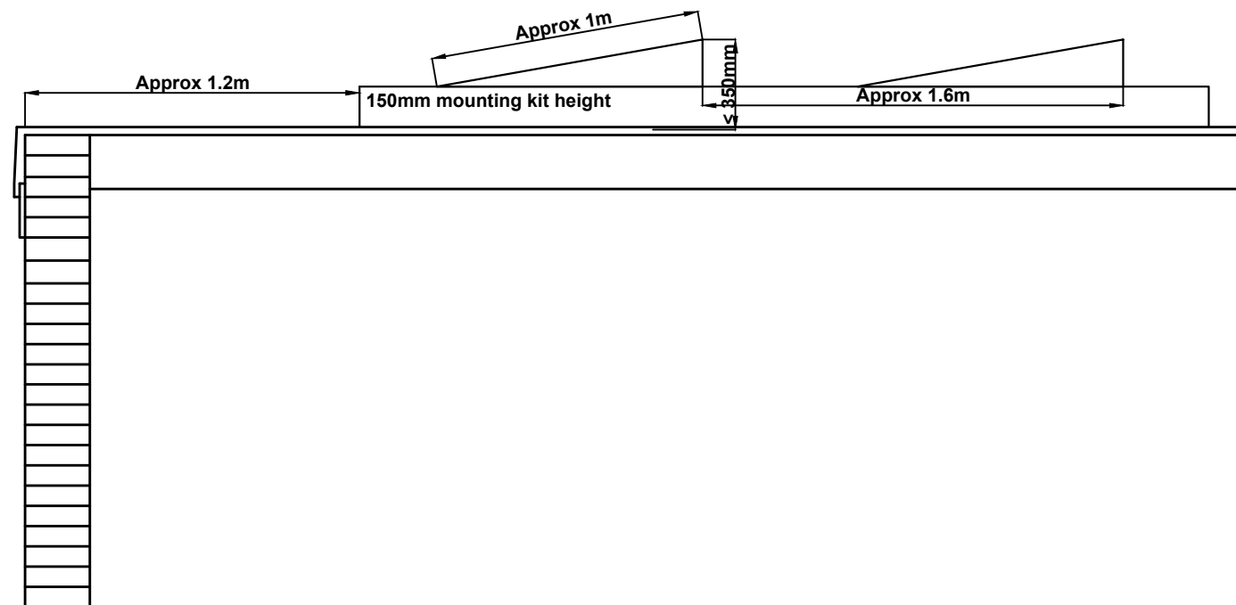
Section A-A 1:25
