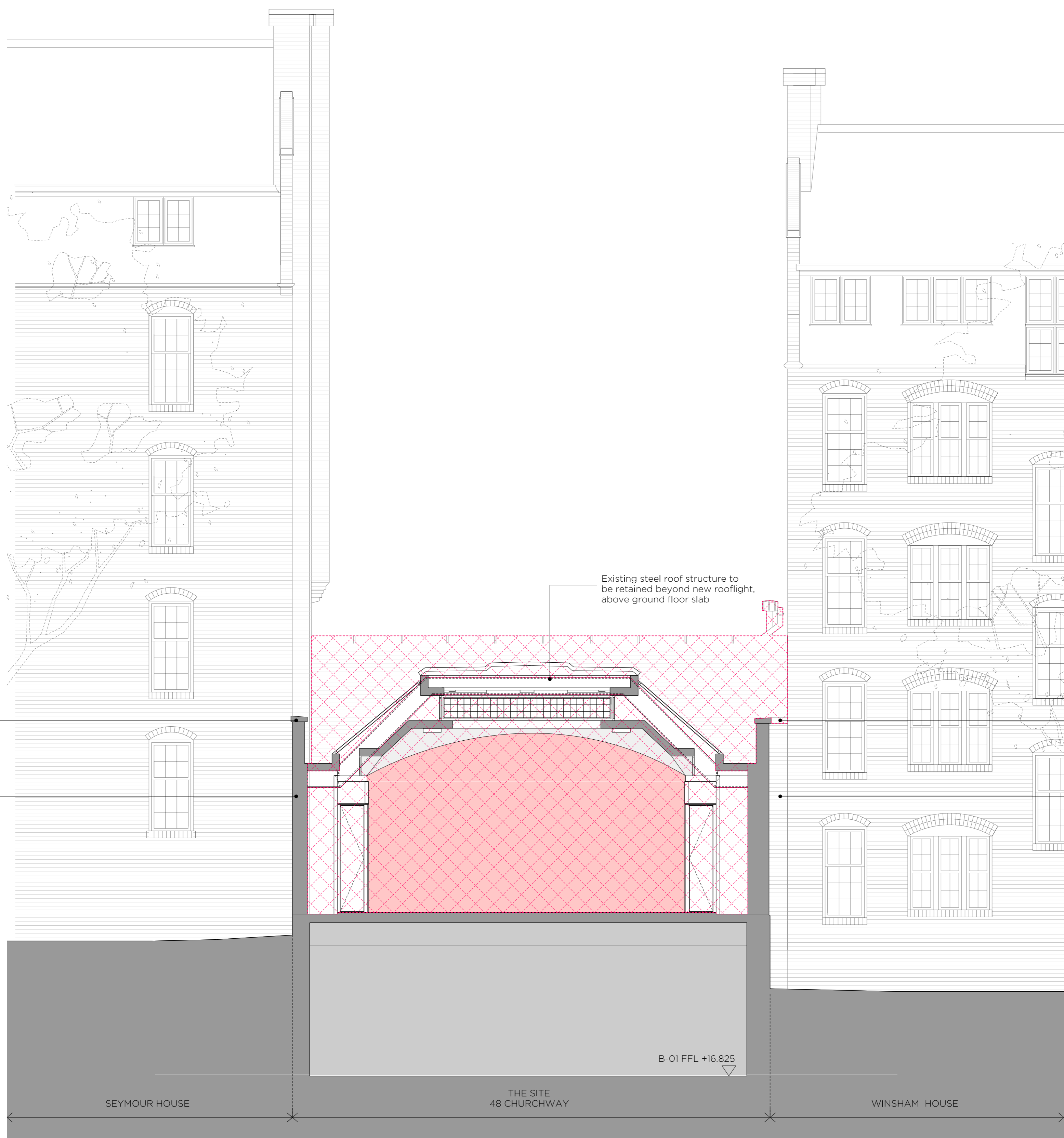
01 SECTION
