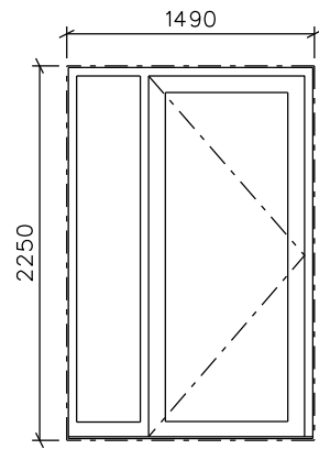
W1 FRONT DOOR inward opening
