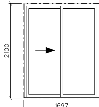
W6 SLIDING DOOR
