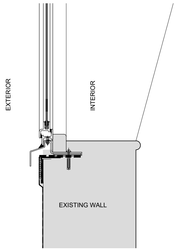
02 Dormer Window Cill Detail- existing 1:5@ A1 / 1:10@ A3
