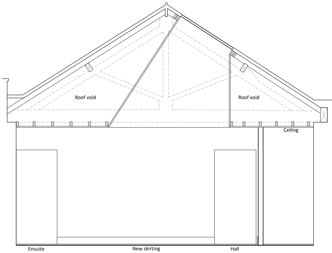
Elevation A
