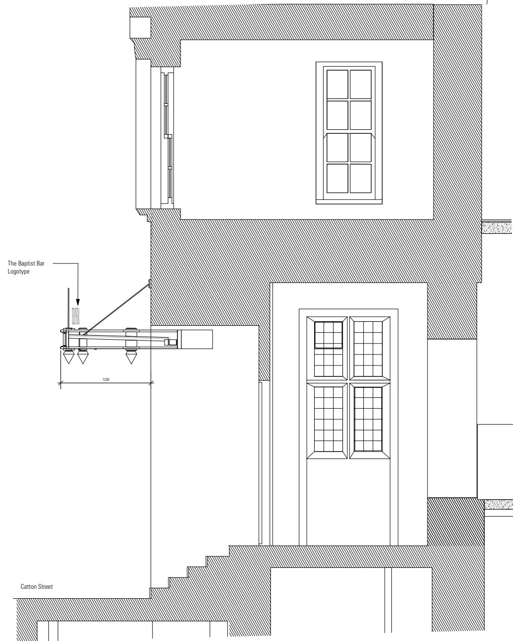
2 Section A-A 1:25@A1, 1:50@A3
