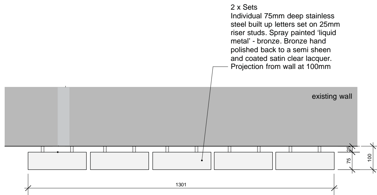
2 Signage Plan 1:10@A3
