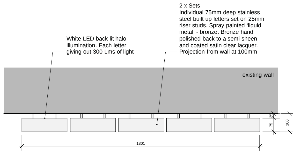
2 Signage Plan 1:10@A3
