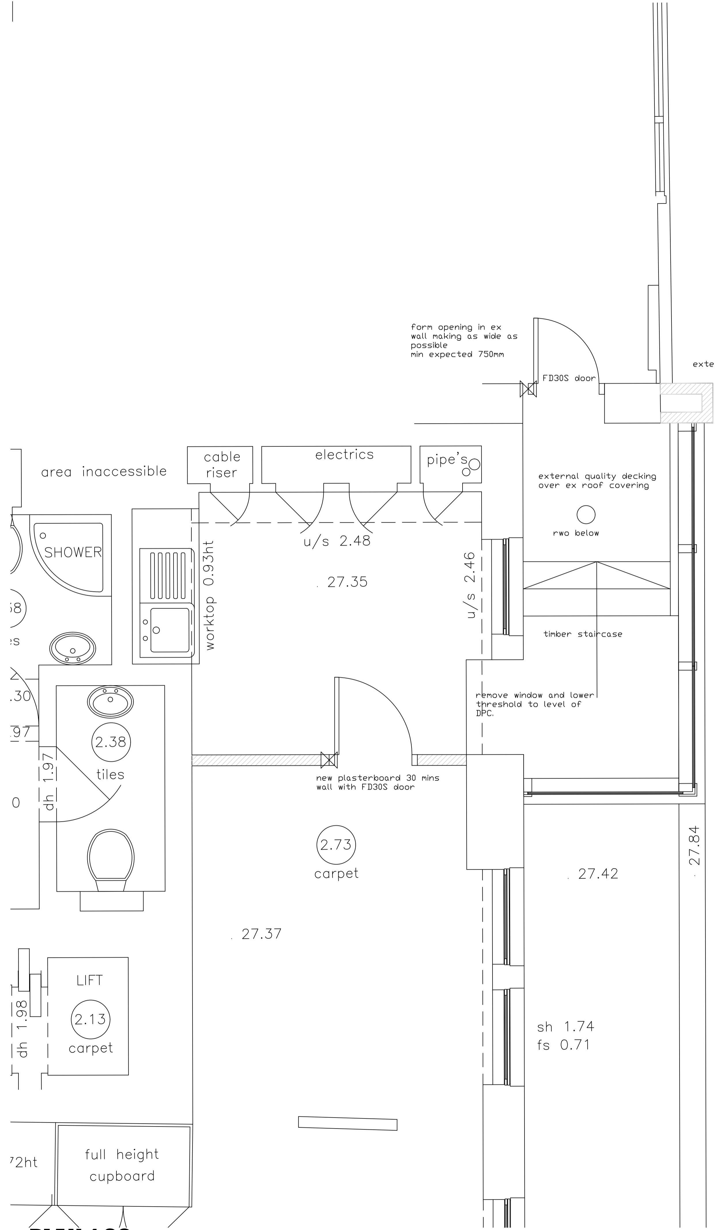
PLAN 1:20
