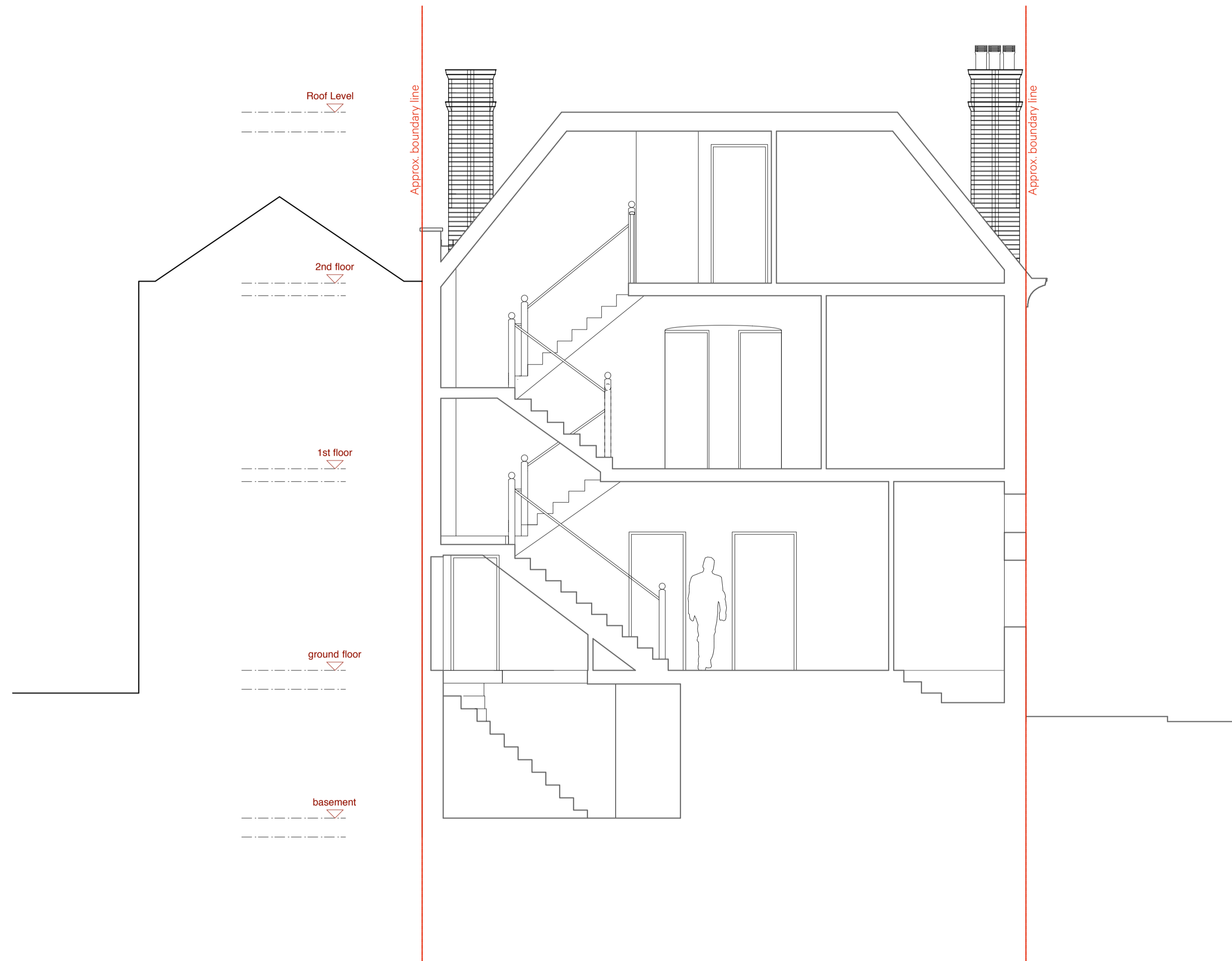
2 Section B-B Scale: 1:50
