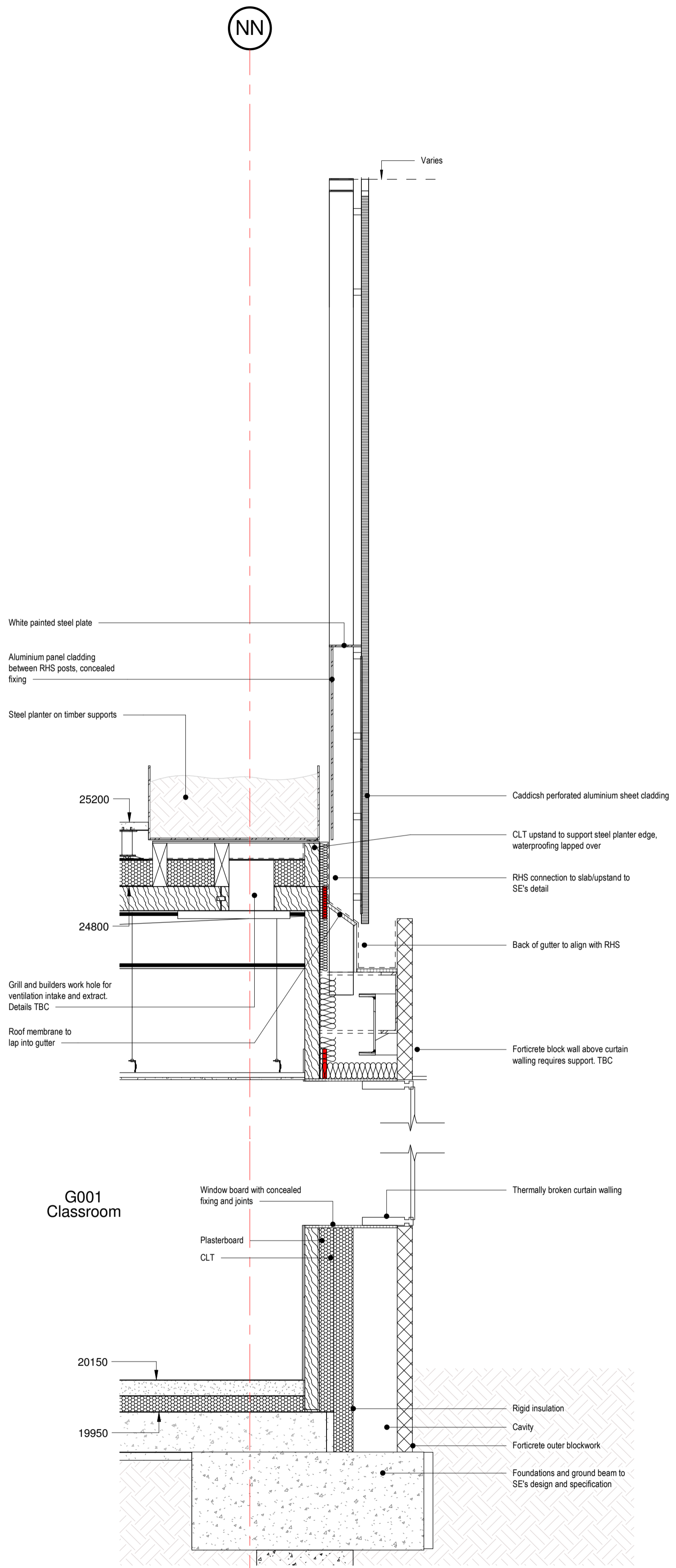
Strip Section 4 1 : 20
