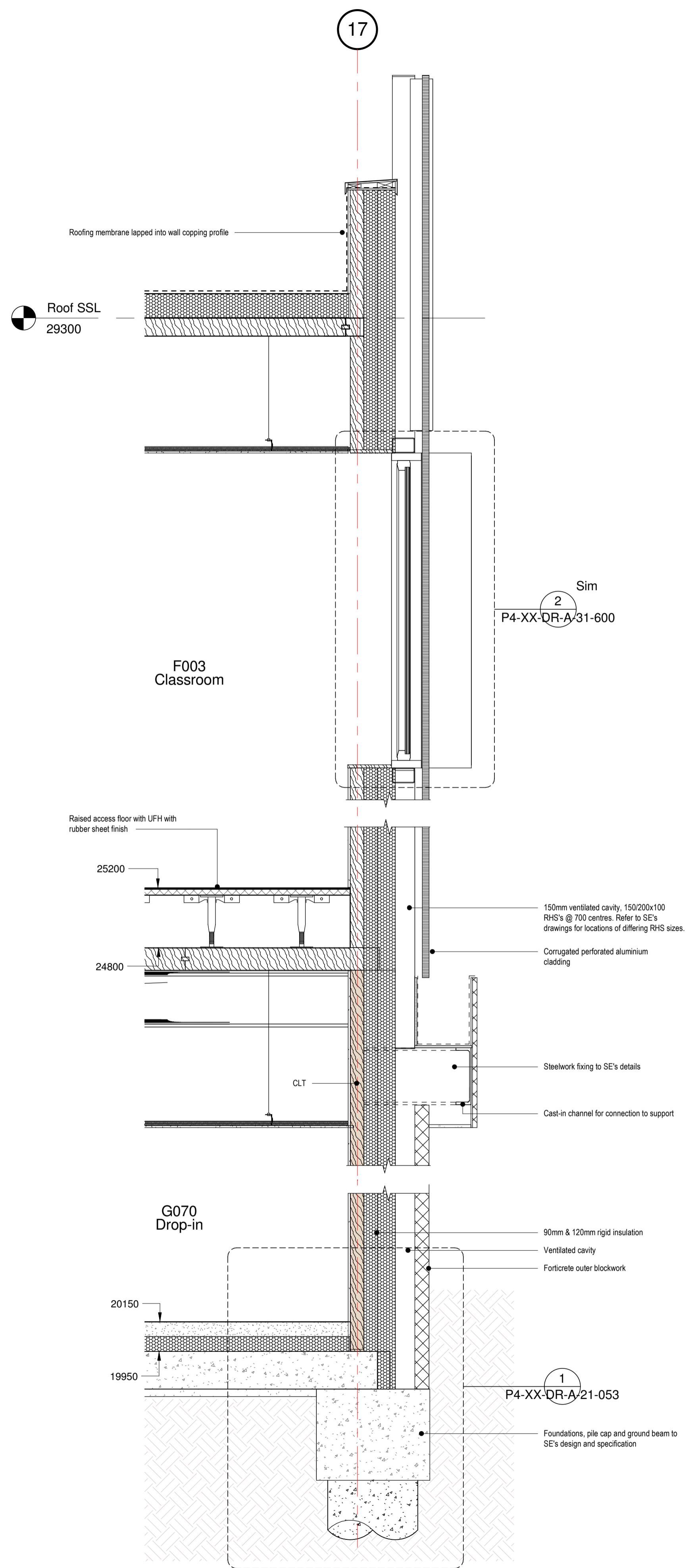
Strip Section 5 1 : 20
