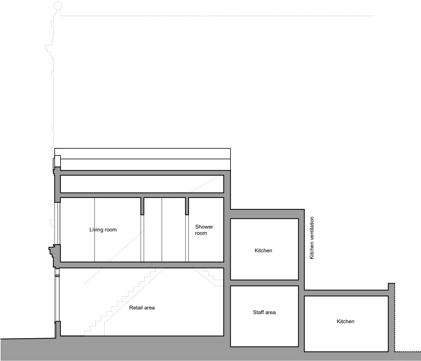
SECTION A-A
