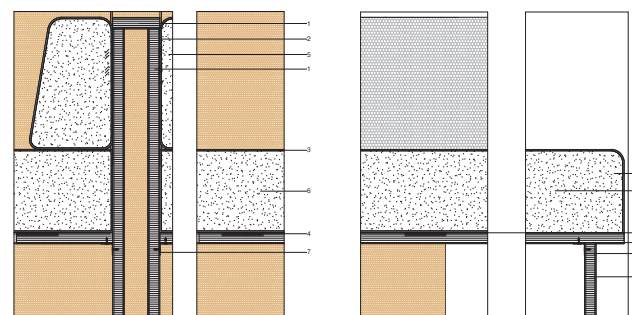
D1 NOOK - BSMNT - DETAIL 1 1:5
