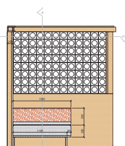
A3 NOOK - BSMNT - SECTION A3 1:20
