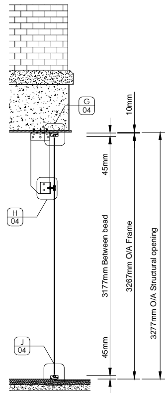
Section View A:A @ 1:50
