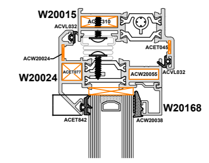
Detail A: Head detail 1:2
