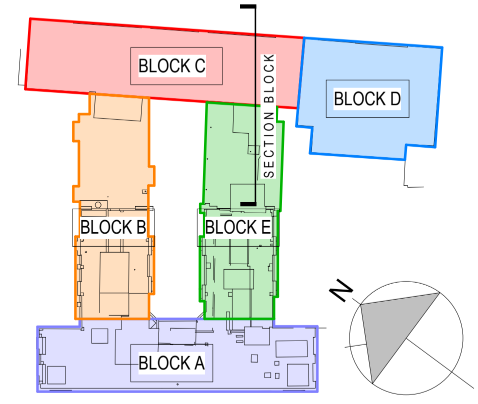
Block Plan 1 : 500
