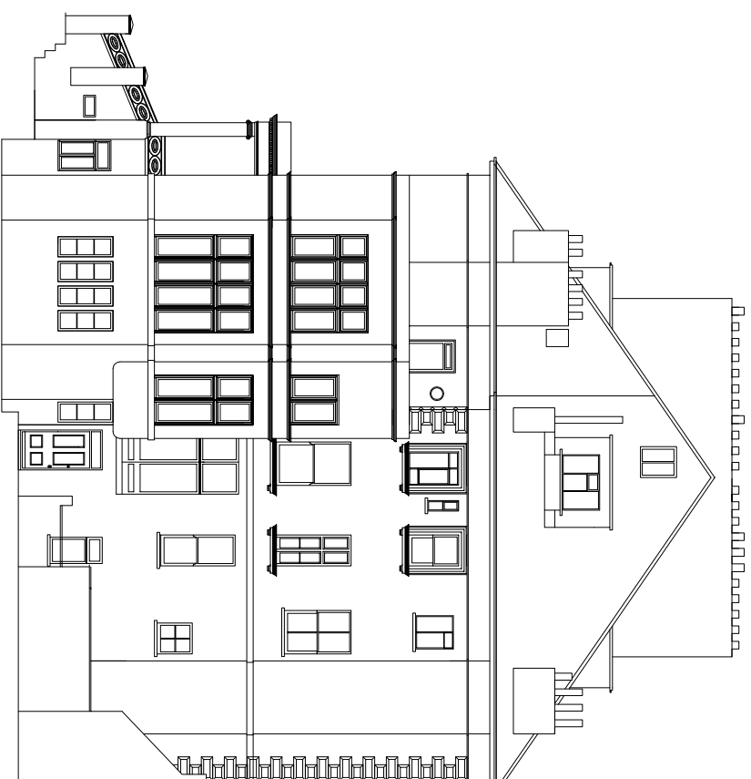
FLANK ELEVATION
