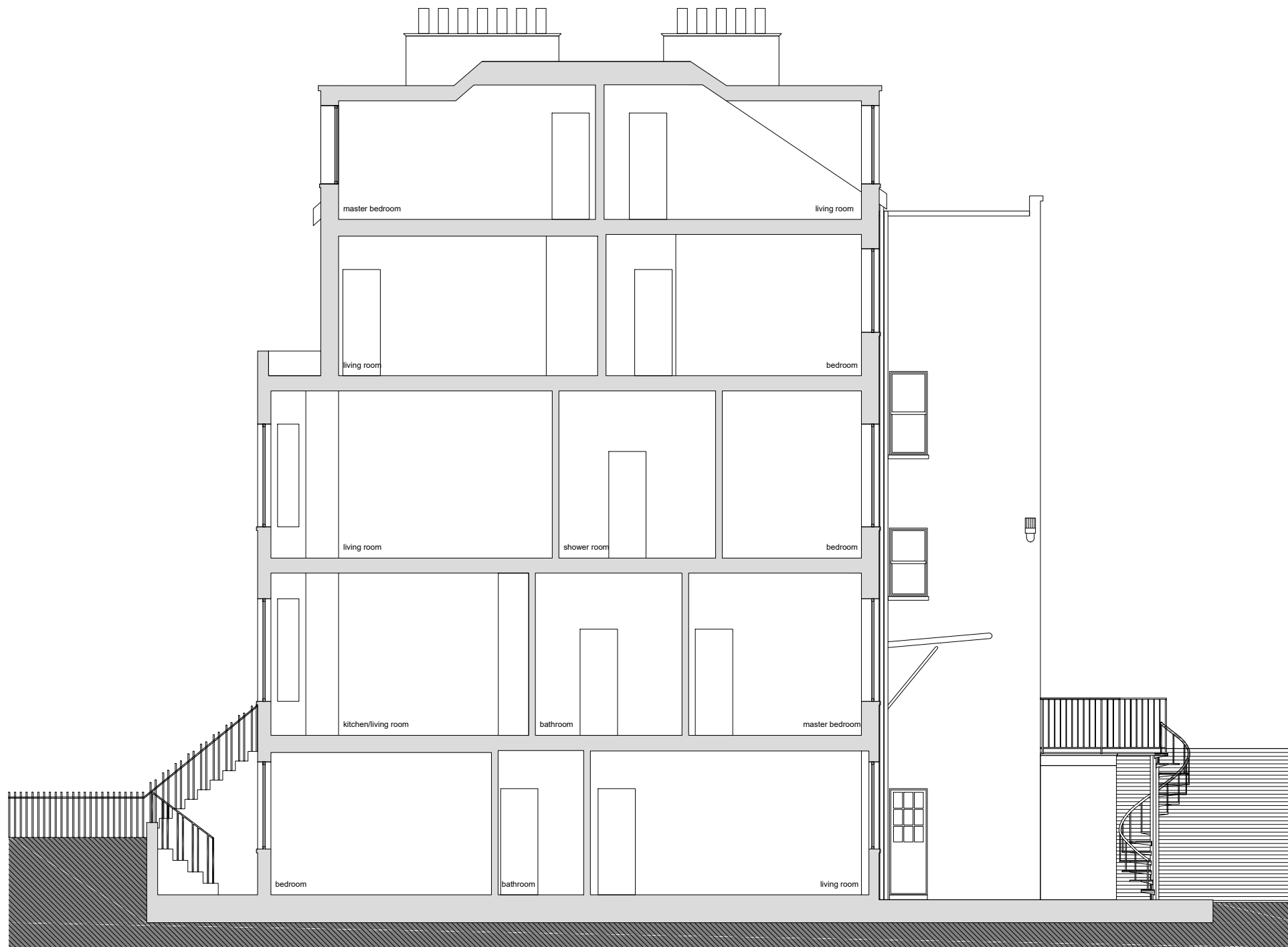
Section DD
