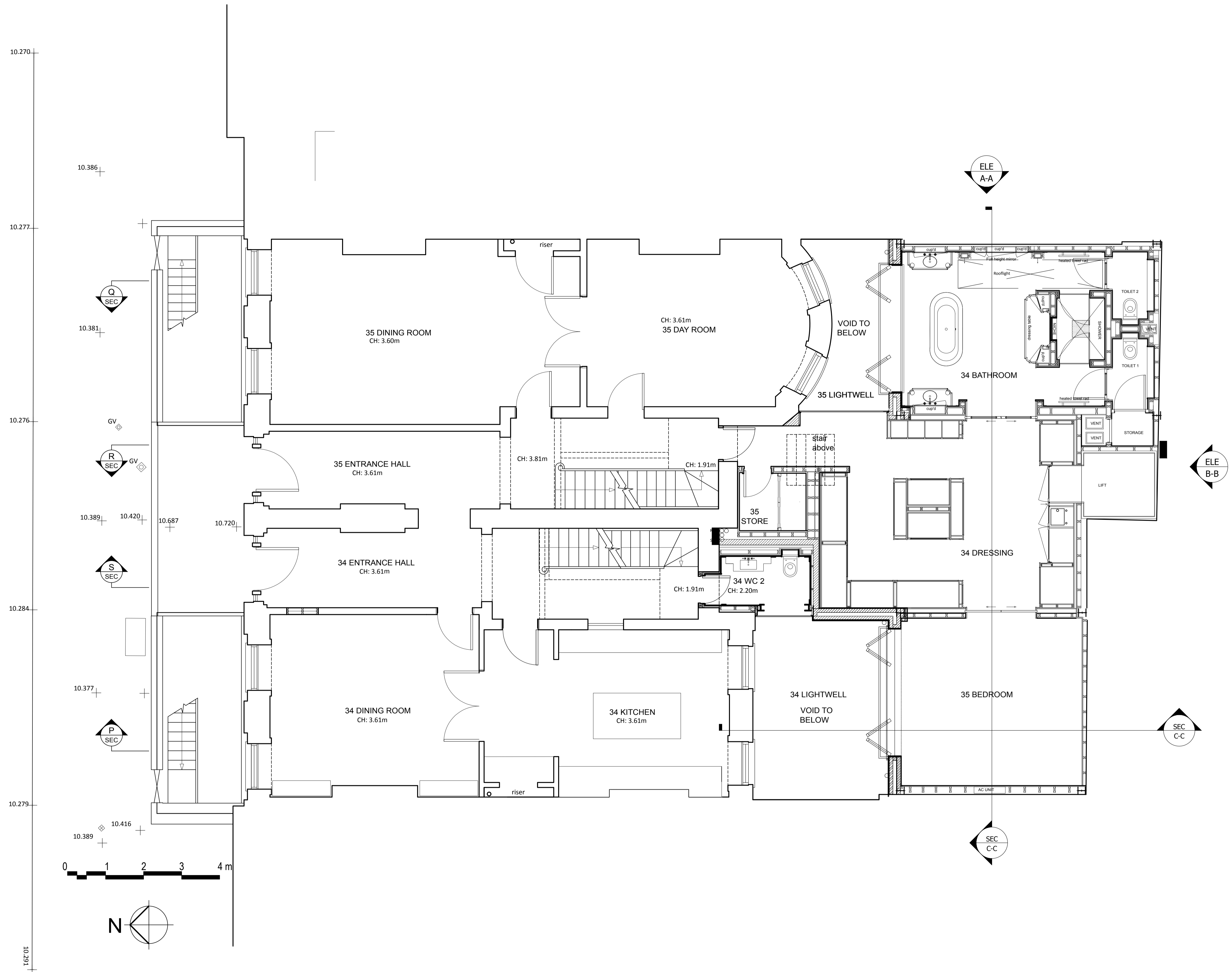
EXISTING PLAN 1:50 @A1 OR 1:100 @A3
