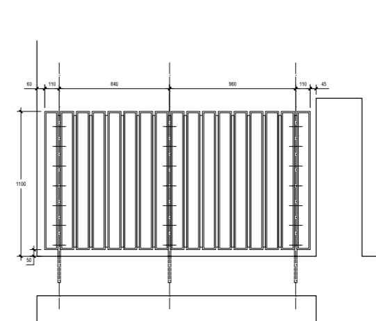
TERRACE E FRONT ELEVATION 6 SCALE: 1:20
