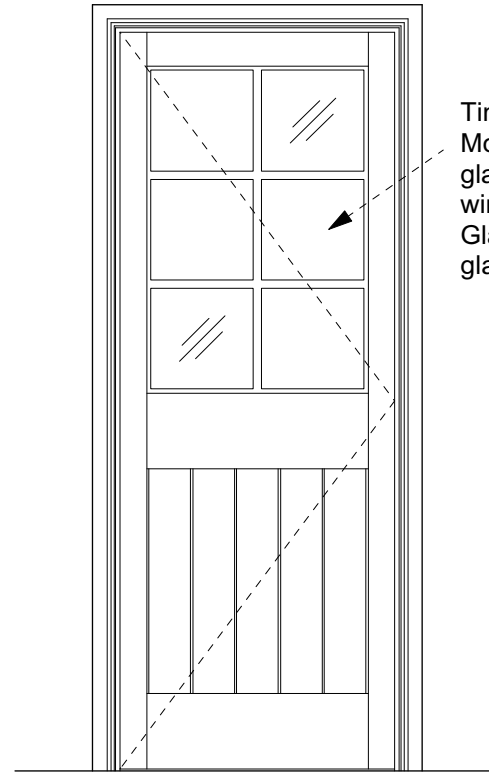
Elevation 1:20
