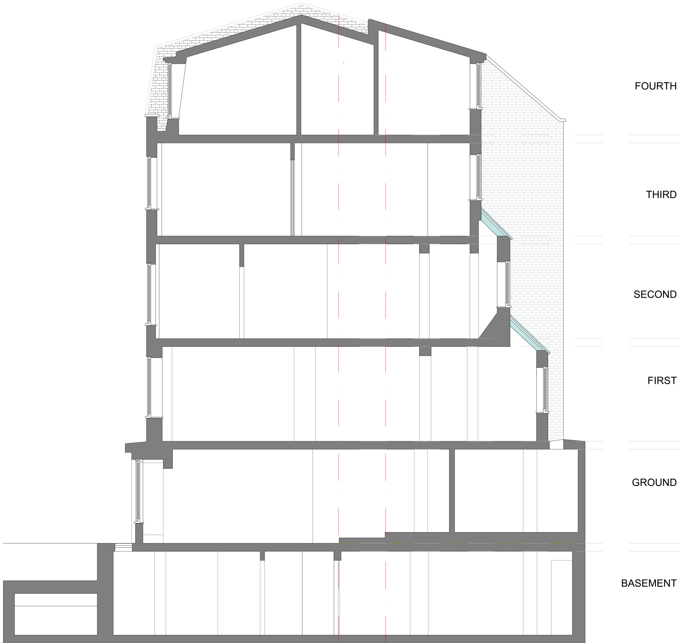
SECTION A-A
