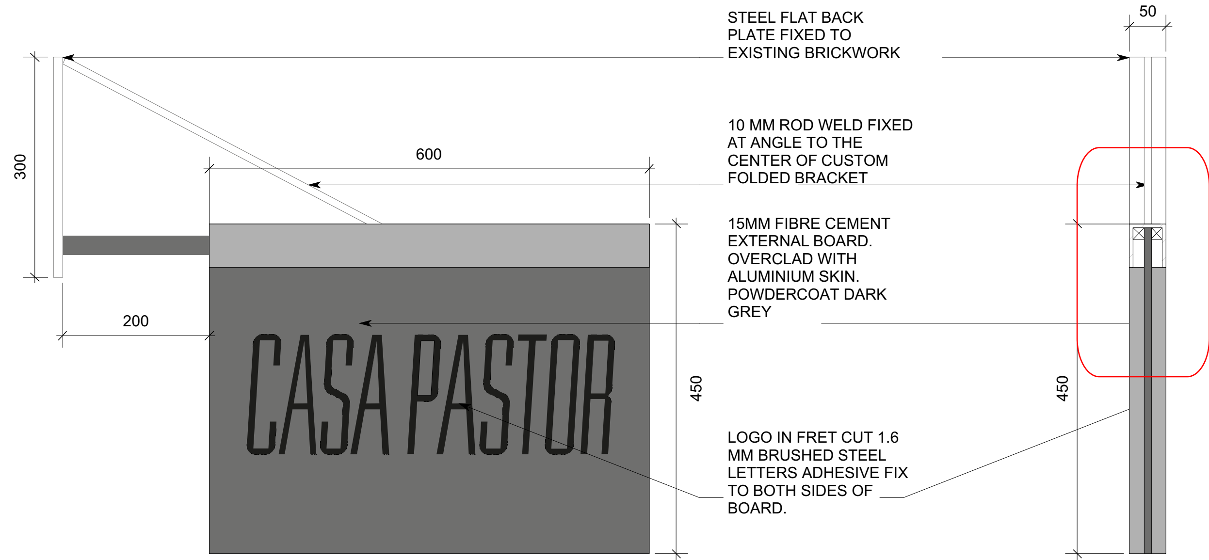
4 Blade Signage Section Scale: 1:5
