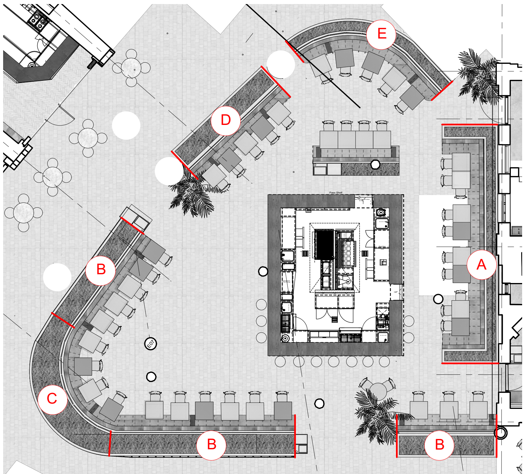
1 Reference Plan Scale: 1:100
