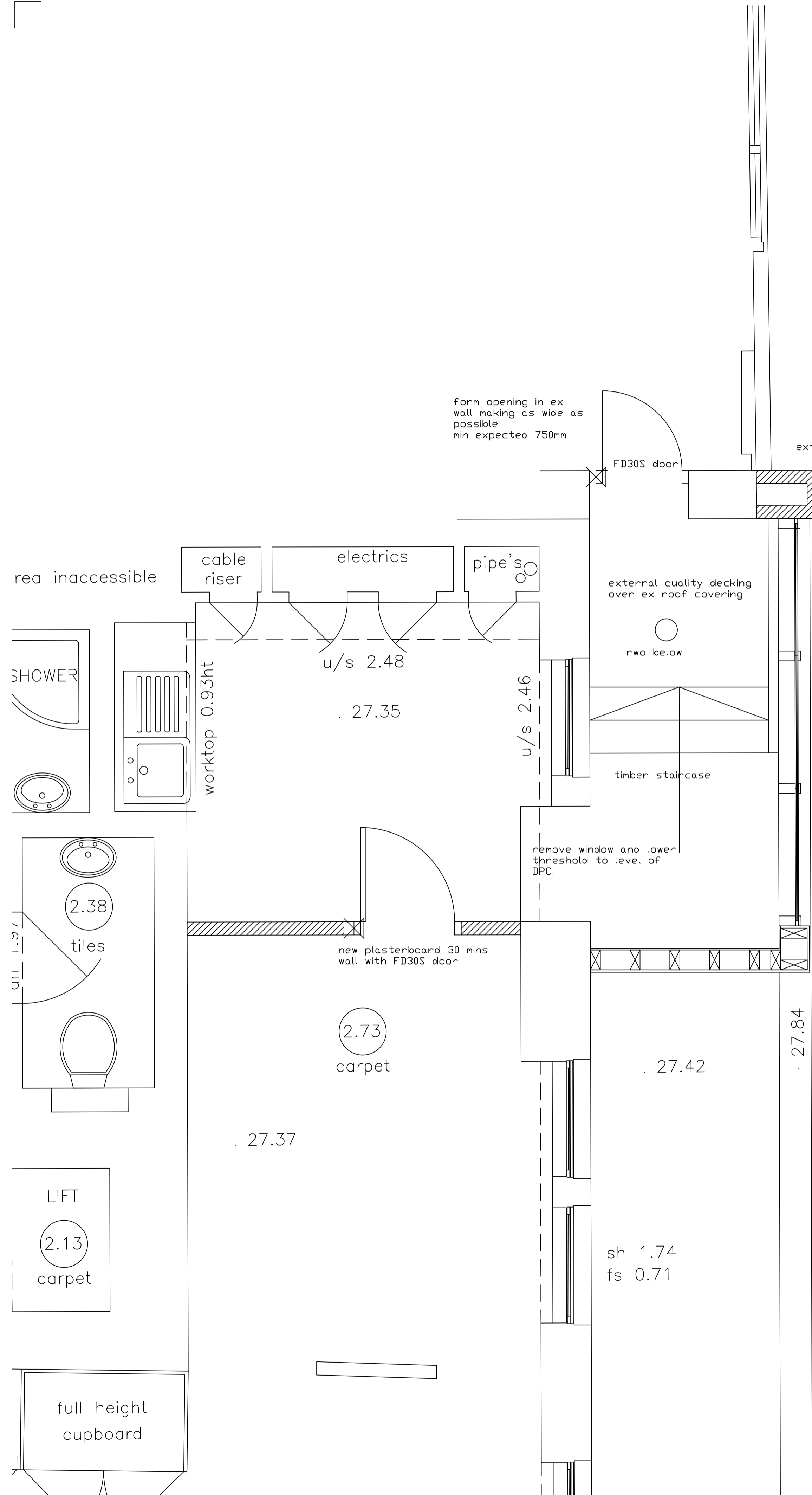
PLAN 1:20
