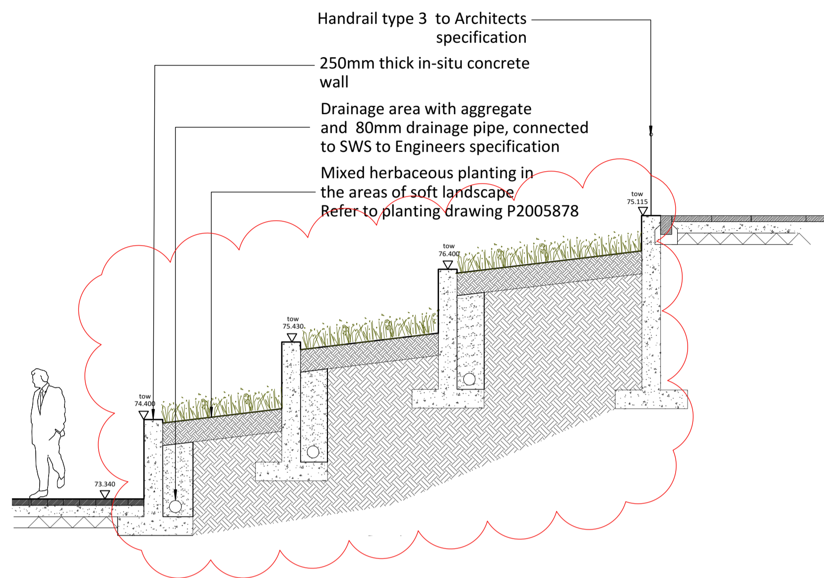
D - SECTION 1:50
