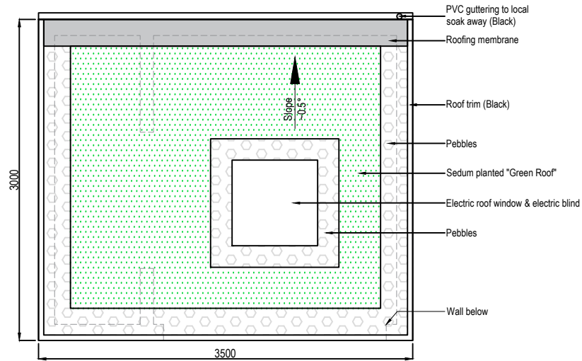
PROP 06 A4 ROOF PLAN SCALE: 1:50@A4
