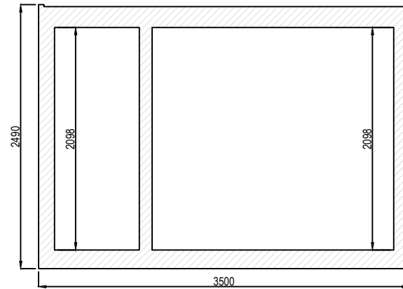
PROP 07 A4 SECTION SCALE: 1:50@A4
