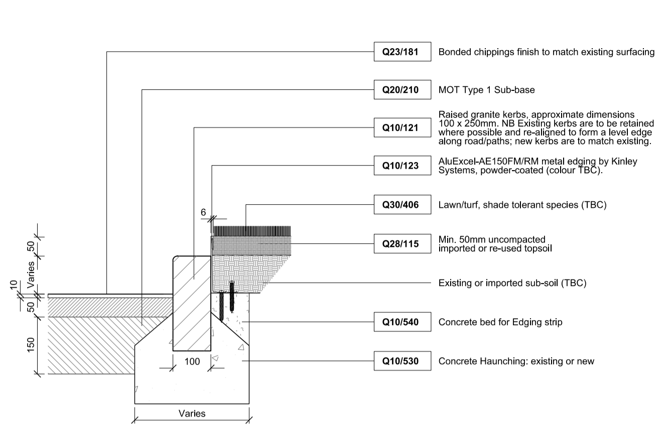
Aluminium Edge/Granite Edge Detail 1
