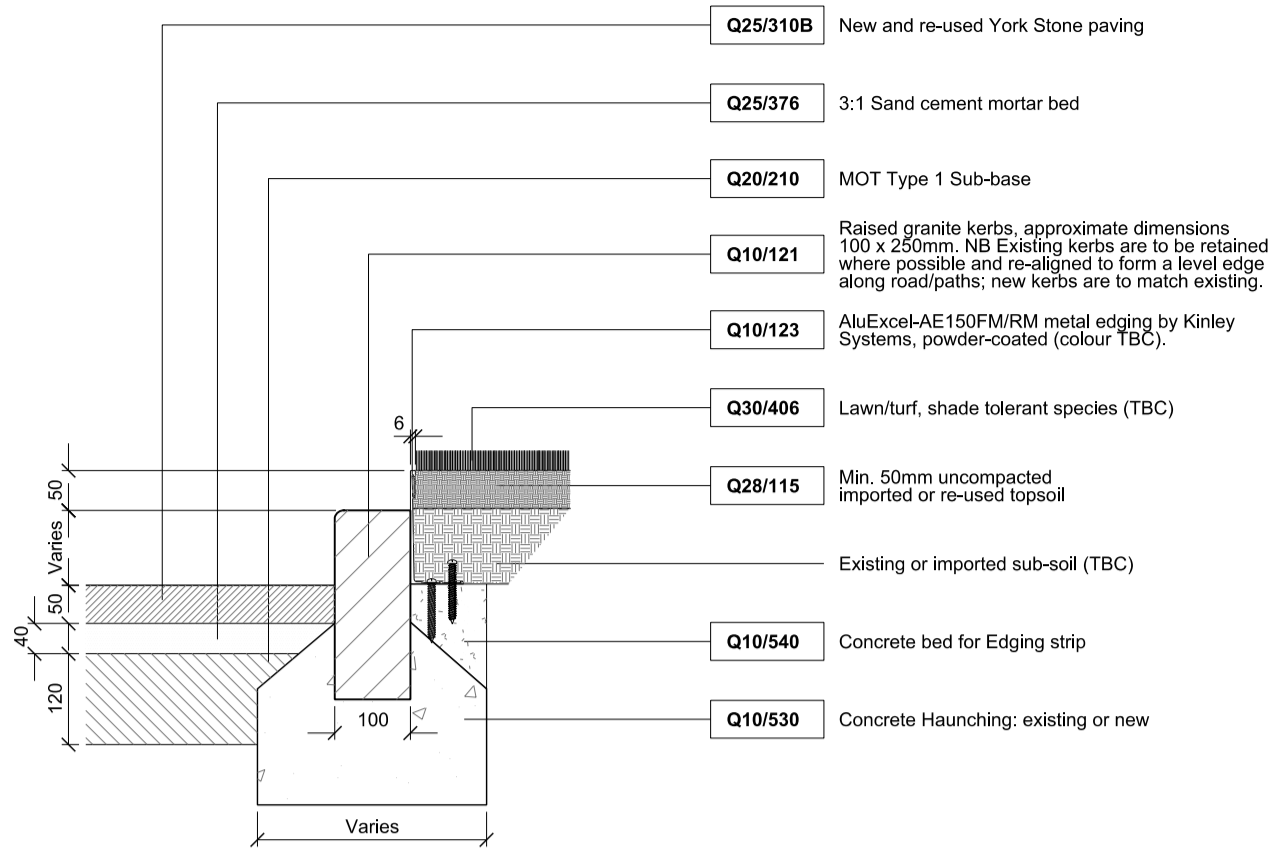
Aluminium Edge/Granite Edge Detail 2
