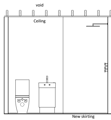
Elevation B
