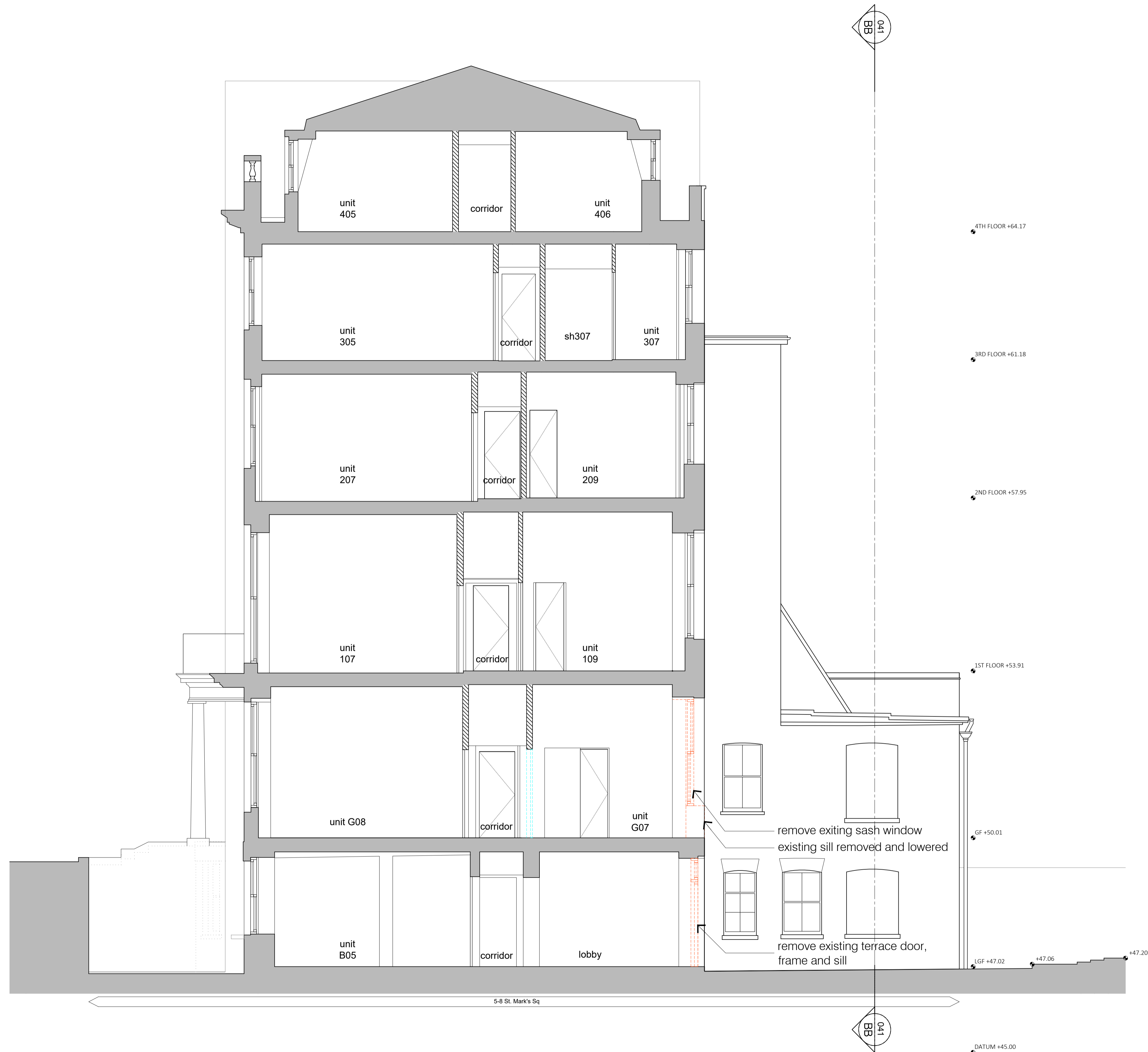
01 Existing section A-A 1:50@ A1 / 1:100 @ A3
