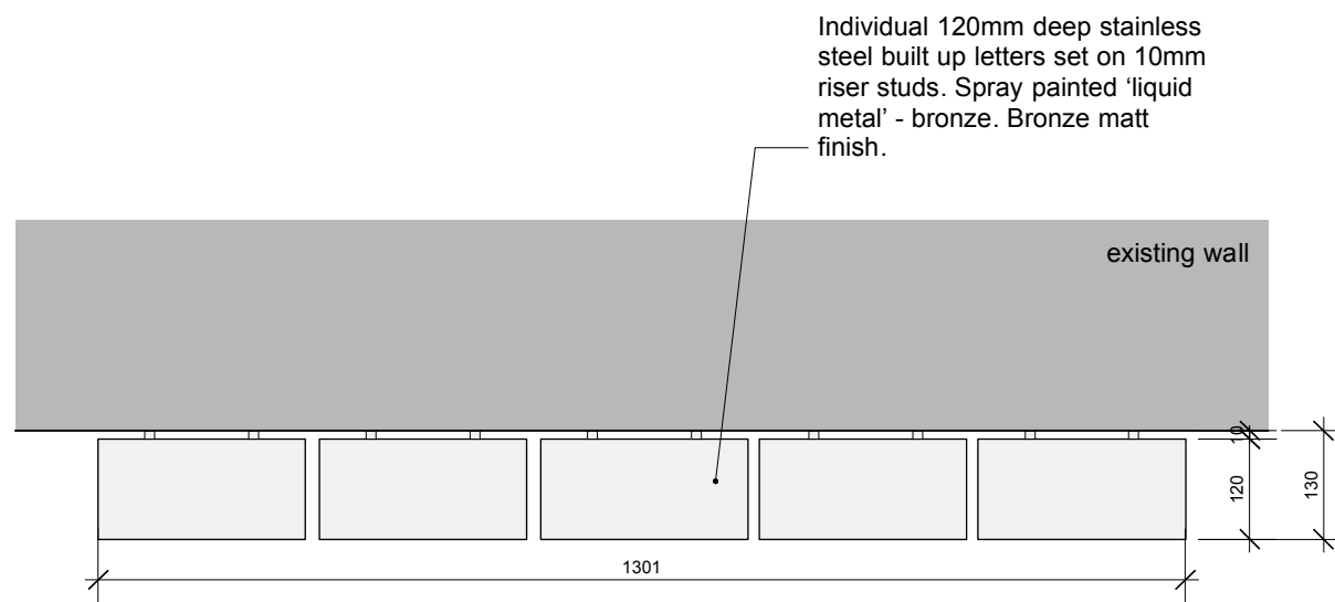
2 Signage Plan 1:10@A3
