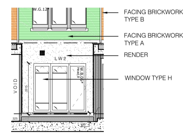
Elevation 2A Scale 1:100
