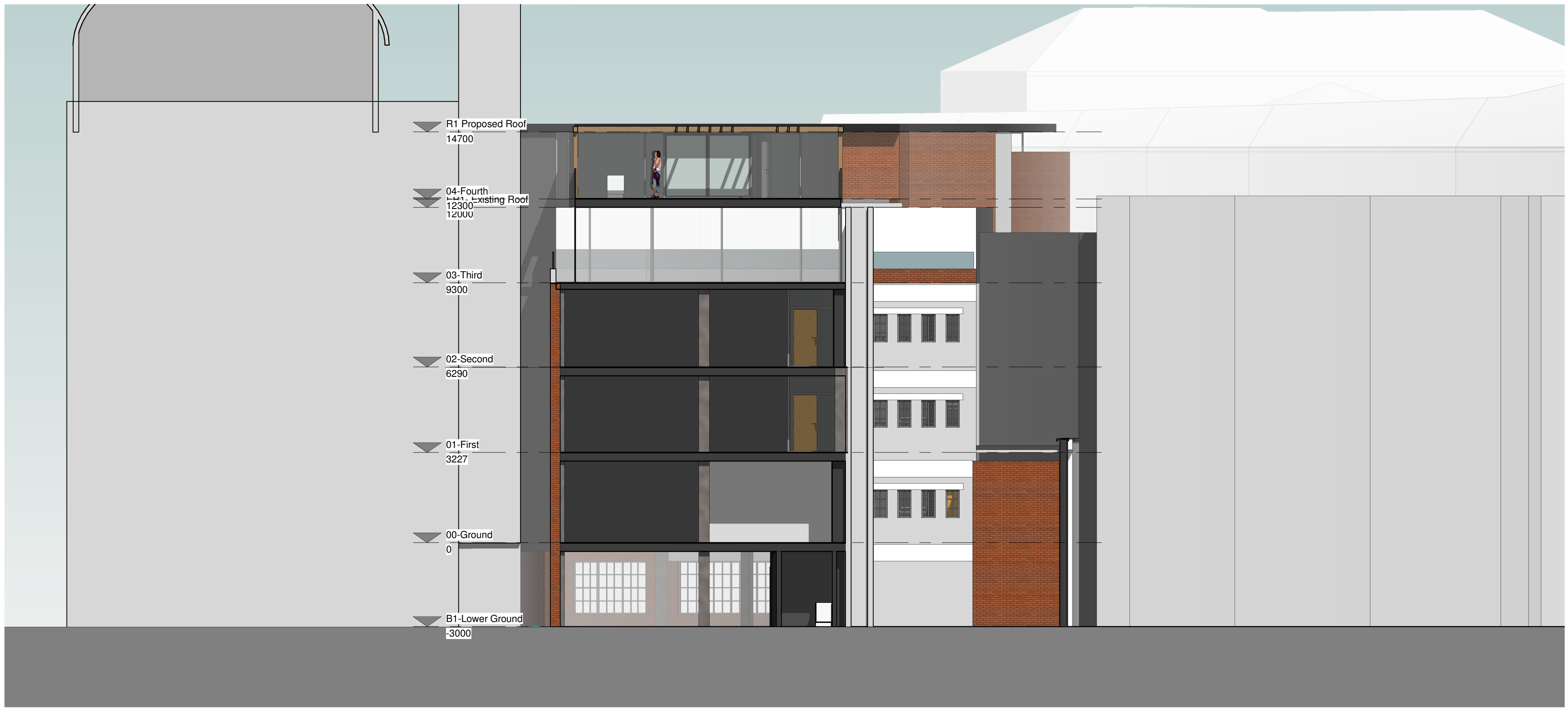
2 Section 3 1 : 100
