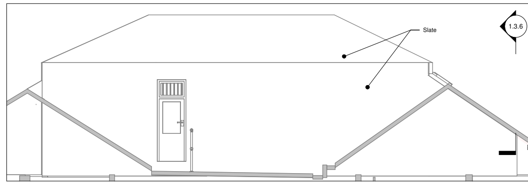
5 Elevation 1.3.5 1 : 50
