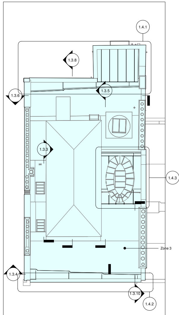
2 Roof Plan 47.06 1 : 100
