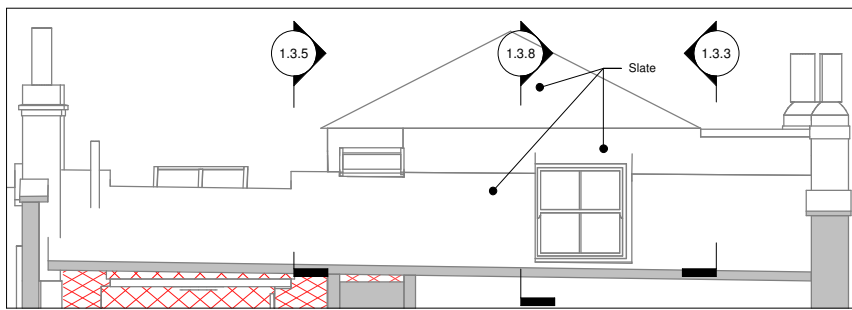
6 Elevation 1.3.6 1 : 50
