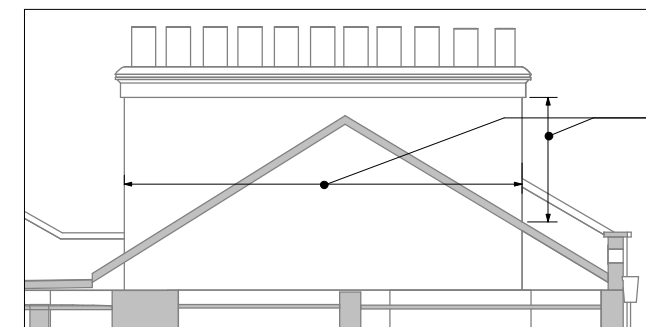
10 Section 1 : 50
