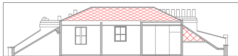
8 Section 1.3.8 1 : 100
