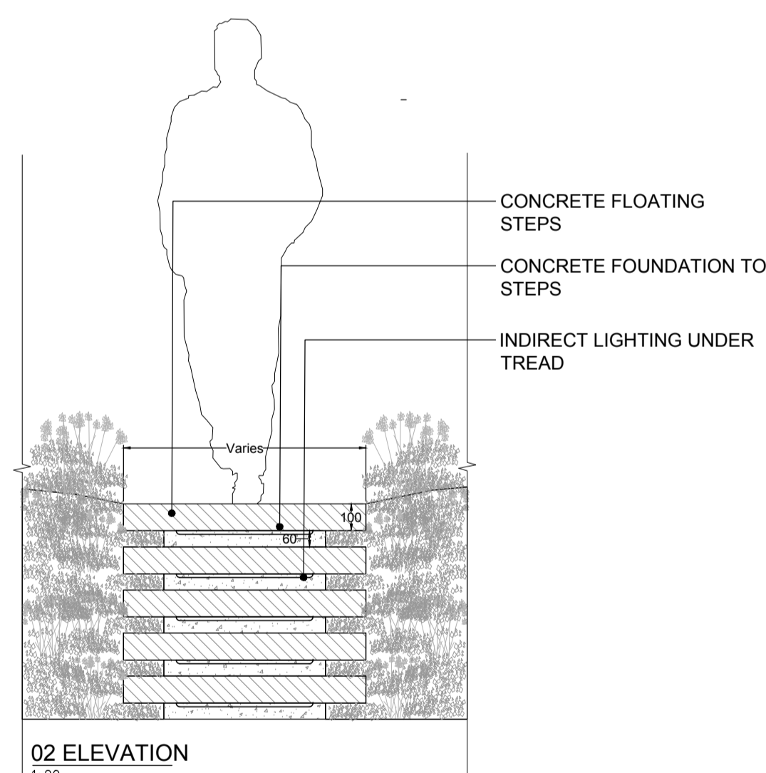
02 ELEVATION 1:20
