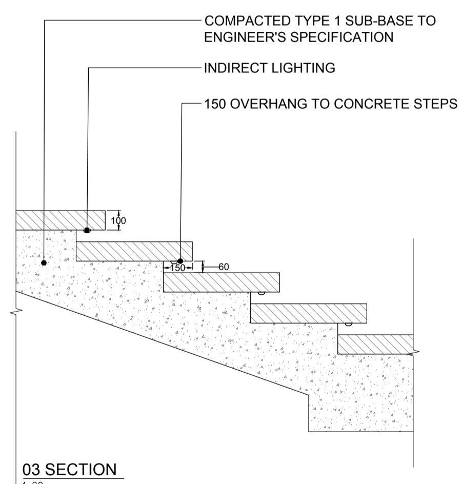
03 SECTION 1:20
