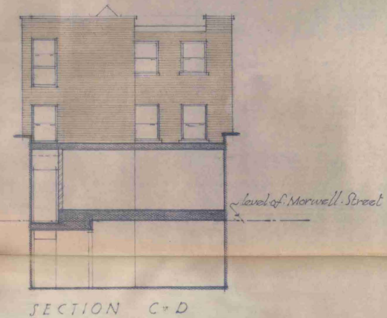
SECTION C-D
